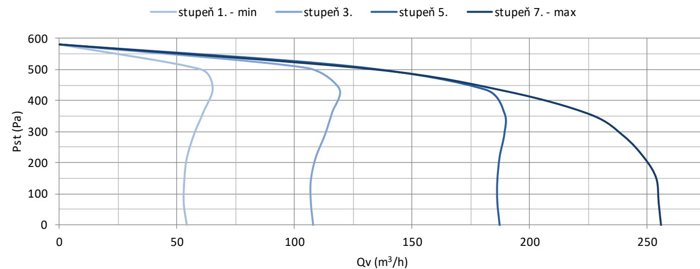
VÝKONOVÉ KŘIVKY - XH2-30-ECS0HRxxS-0A0
